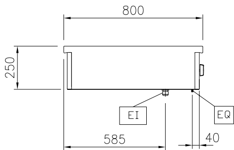
Zij aanzicht
